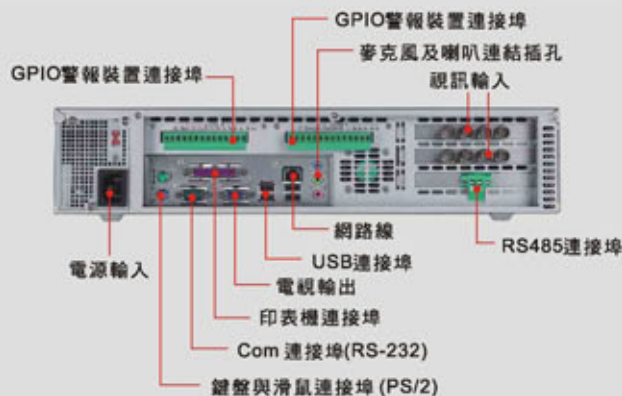
背面板
